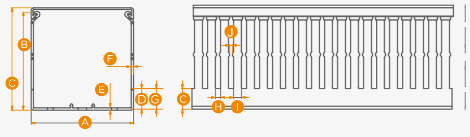
Kablo Kanalı
